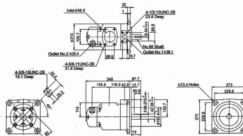
SQP42 法兰安装尺寸
