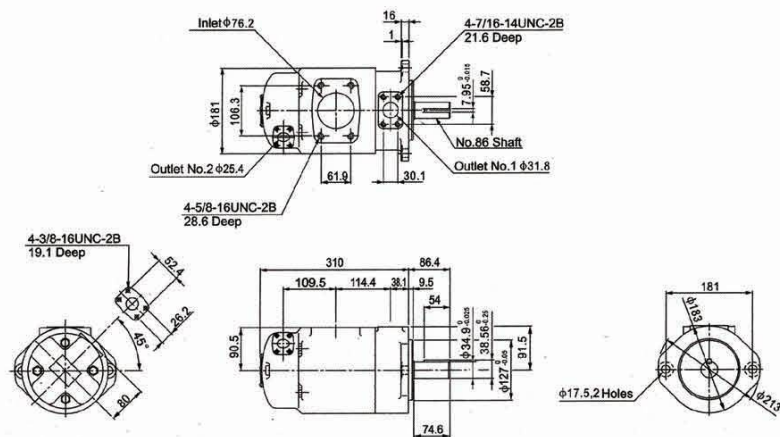
SQP32 法兰安装尺寸
