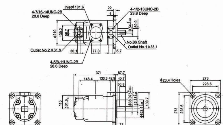
SQP43 法兰安装尺寸
