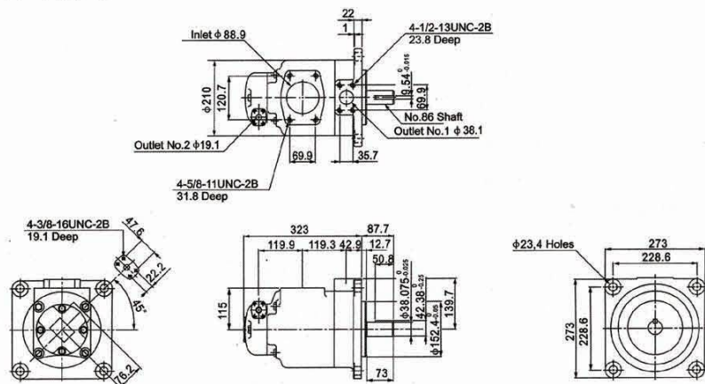
SQP41 法兰安装尺寸
