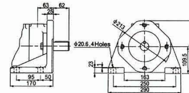
SQP3 脚座安装尺寸
