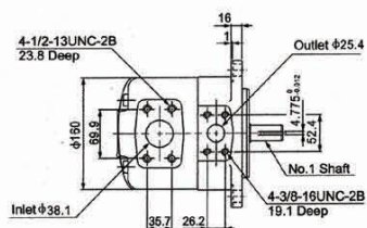
SQP2 法兰安装尺寸
