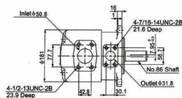
SQP3 法兰安装尺寸
