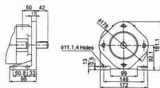
SQP1 脚座安装尺寸
