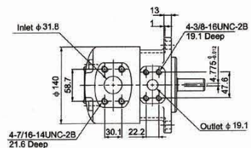
SQP1 法兰安装尺寸
