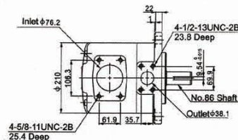
SQP4 法兰安装尺寸
