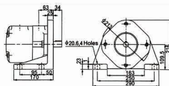
SQP2 脚座安装尺寸
