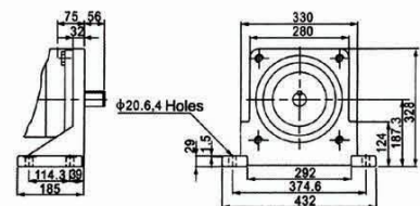
SQP4 脚座安装尺寸
